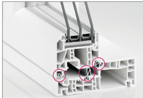
Tre omløbende tætningsniveauer
